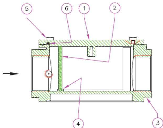
FM DN32÷DN50
