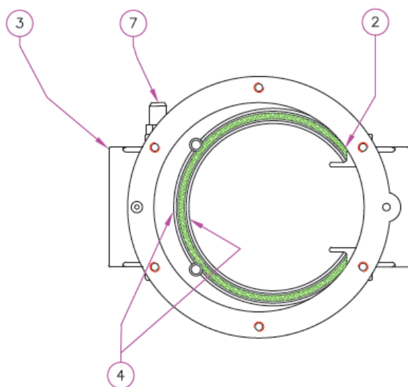
FM DN65÷DN80
