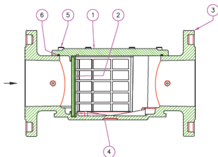
FM DN65÷DN80
