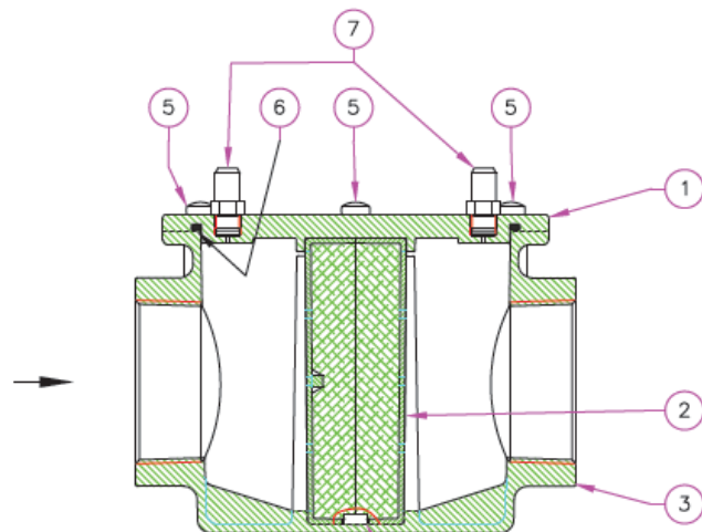
FGM DN32÷DN50
